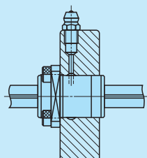
法兰型安装示例 (油孔/OH规格)
