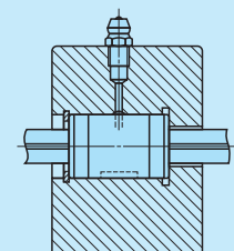
标准型安装示例 (油孔/OH规格)
