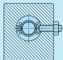
大小尺寸为2、3、4的外筒止转
