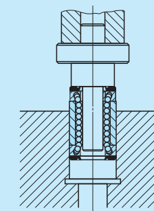
图3 外筒的压入方法
